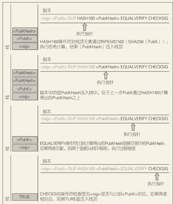
图 5.4 评估一个P2PKH交易的脚本 (第2部分)
